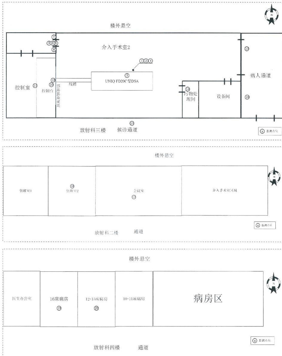
图1 UNIQ FD20C型 DSA 应用场所监测点位布置图 (DSA 状态)
