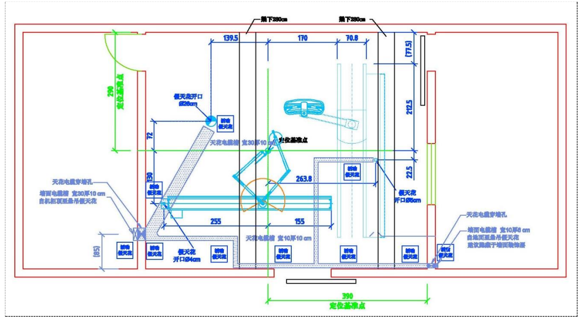
图 2-6 9 号楼三楼放射科介入室 2 电缆沟设计图
