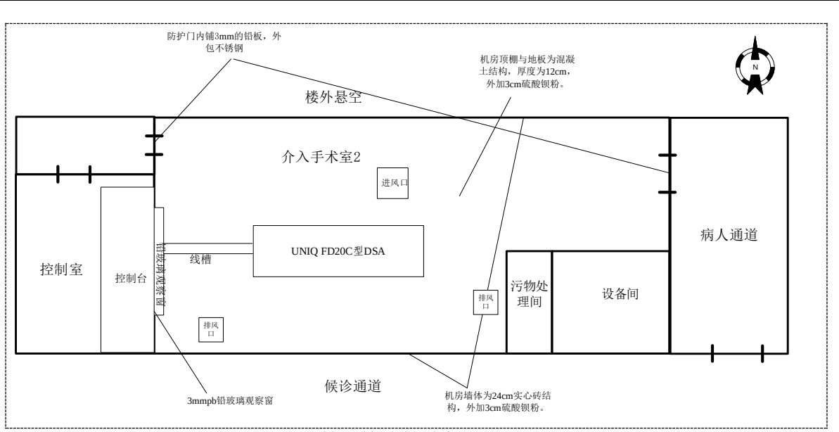
图 2-5 9 号楼三楼放射科介入室 2 平面防护图
