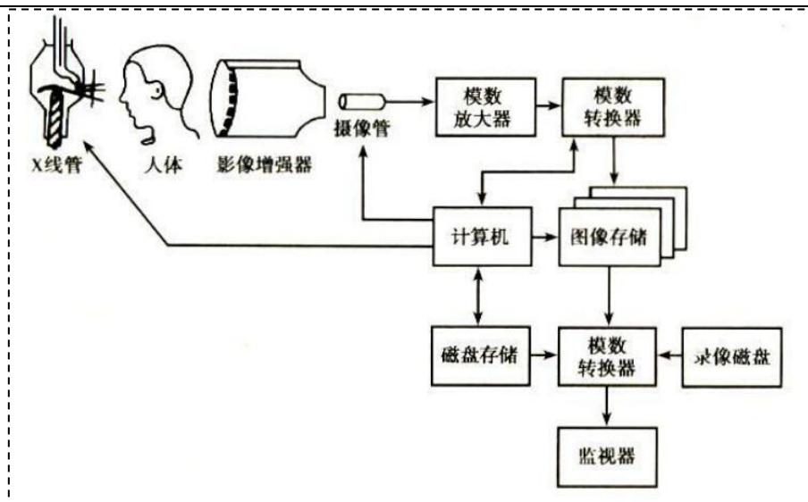
图 2-7 DSA 基本结构图
